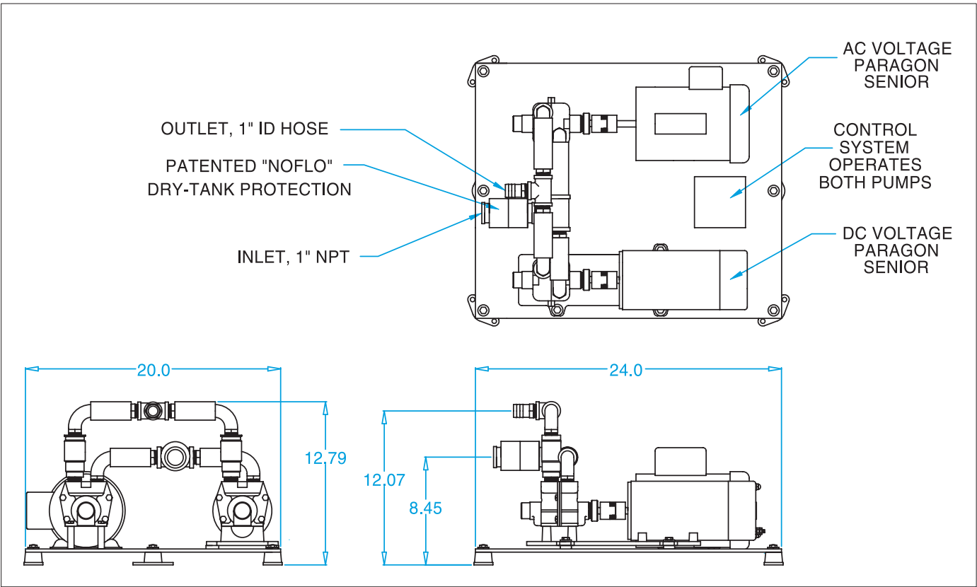
PAR DIMENSIONS
